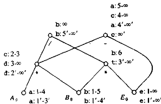
Fig. 10.69. Annotated dag.
