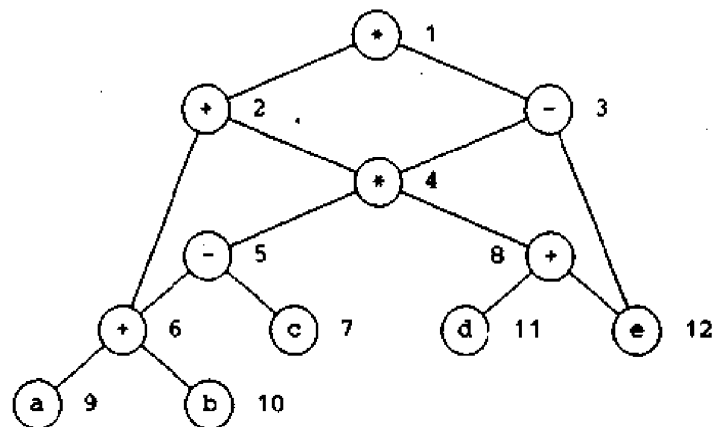
Fig. 9.22. A dag.
