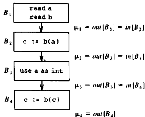
Fig. 10.66. Example program.
