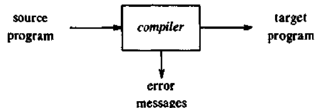
Fig. 1.1. A compiler.
