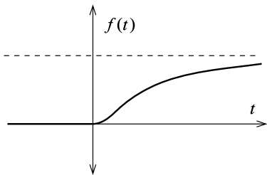
Fig. 2.4 f(t) = e^{-1/t}
