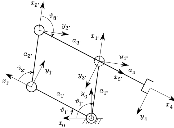
Fig. 2.21. Parallelogram arm
