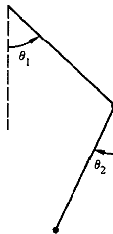
FIGURE 1.4 Double pendulum.
