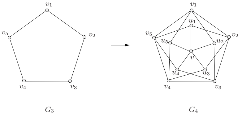
Fig. 14.6. Mycielski's construction
