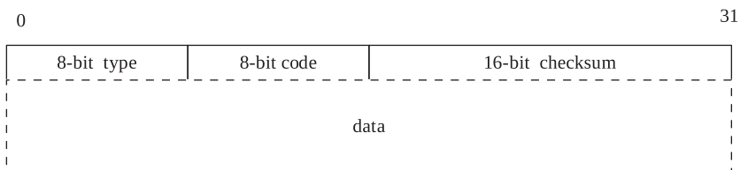
Figure 2.35b. ICMP message format.
