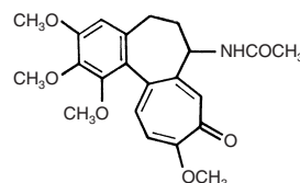
COLCHICINE
