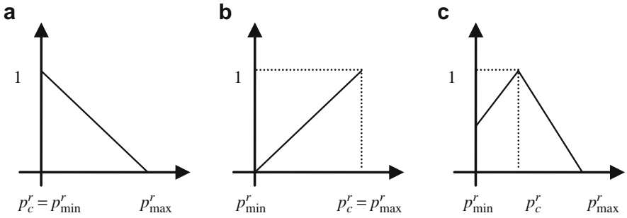
Fig. 3.2 P^r(i) function
