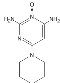
Minoxidil
