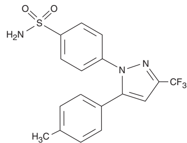
Celecoxib
