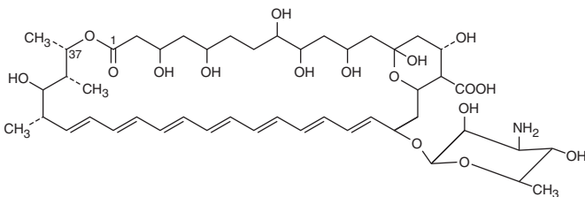
Amphotericin B
