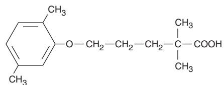
Gemfibrozil
