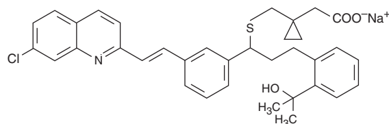
Montelukast
