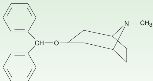
Benztropine
