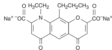
Nedocromil sodium
