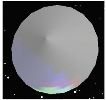
Cone
