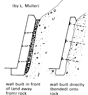
16 The Ebensee Krainer wall
