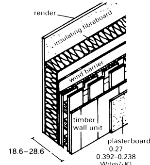
14 Timber unit wall (Lignotrend)
