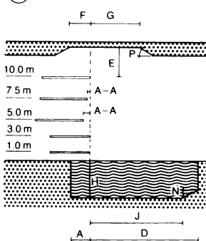
8 Longitudinal section
