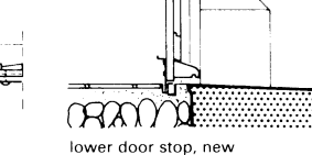
lower door stop, new
