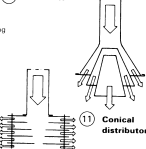
12 Air distribution fins
