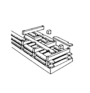
16 The Ebensee Krainer wall
