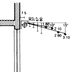
⑲ Adjustable awning
