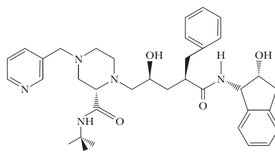
Crixivan (indinavir)
