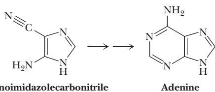
Aminoimidazolecarbonitrile
