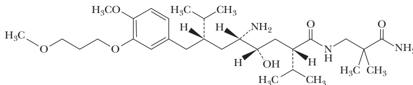
Aliskiren
