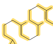
Phytol
